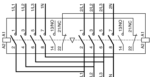
电源转切接触器组，带有集成的电气互锁装置 (LAD9R1V)
