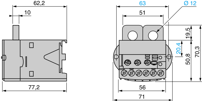
LT47●●●●
