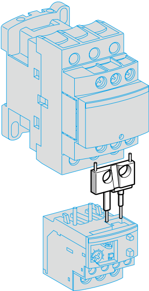
LAD7C●
