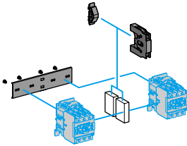
LA9D4002
