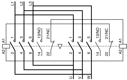
电源转切接触器组，带有集成的电气互锁装置 (LAD9R1V)
