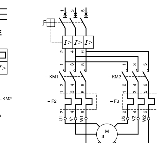
部分绕组电动机 GV2LE
